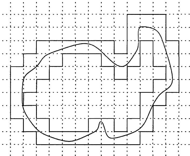
图 2.2 集合内含量和外含量的近似。
