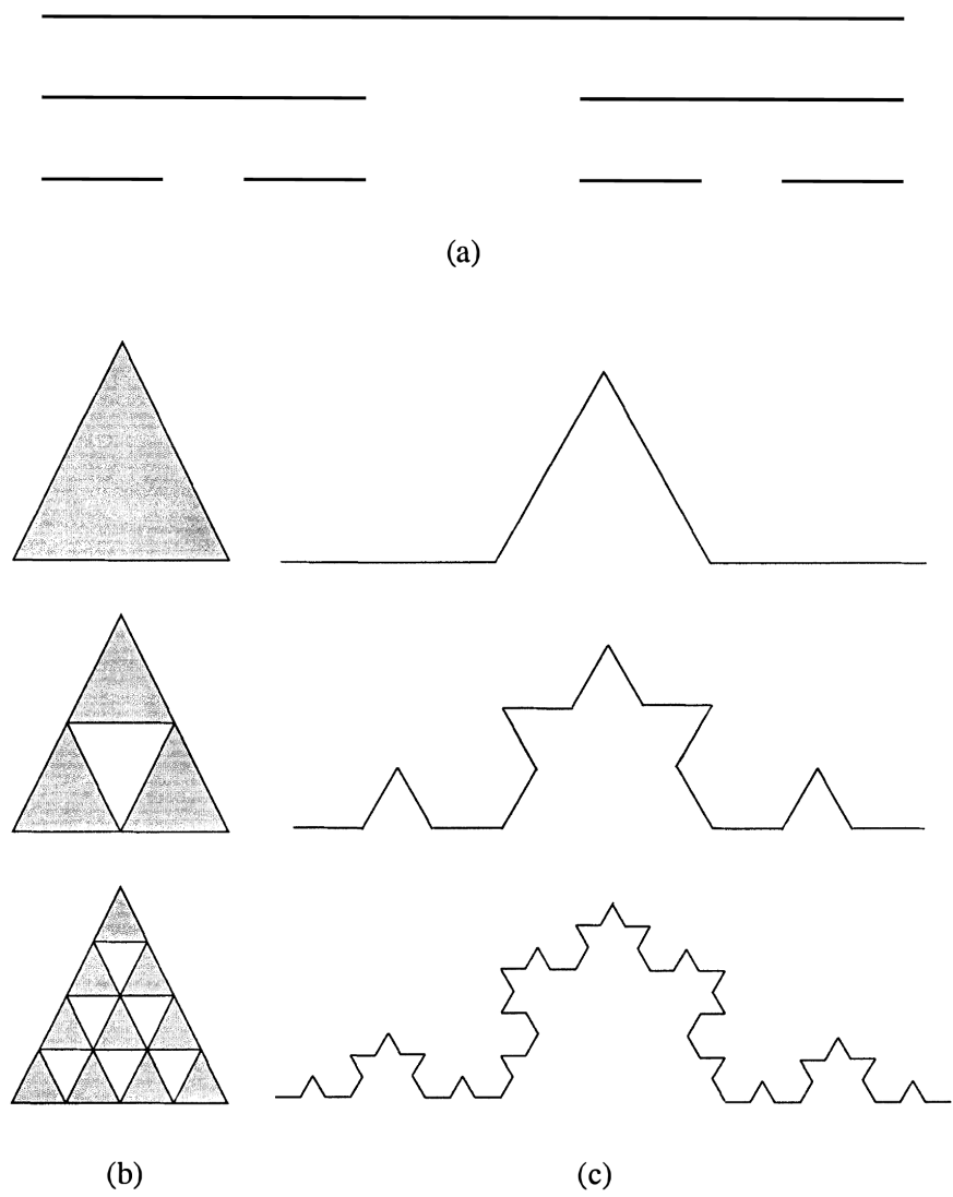
图 11.1 (a) Cantor 集 C_{3/8} 、(b) Sierpiński 垫片和 (c) 雪花曲线的前三次近似。
