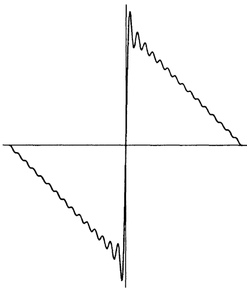
图 8.1 Gibbs 现象: 函数 y = \sum_{k=1}^{30} (\pi k)^{-1} \sin 2\pi kx , -\frac{1}{2} \leq x \leq \frac{1}{2} 的图像。
